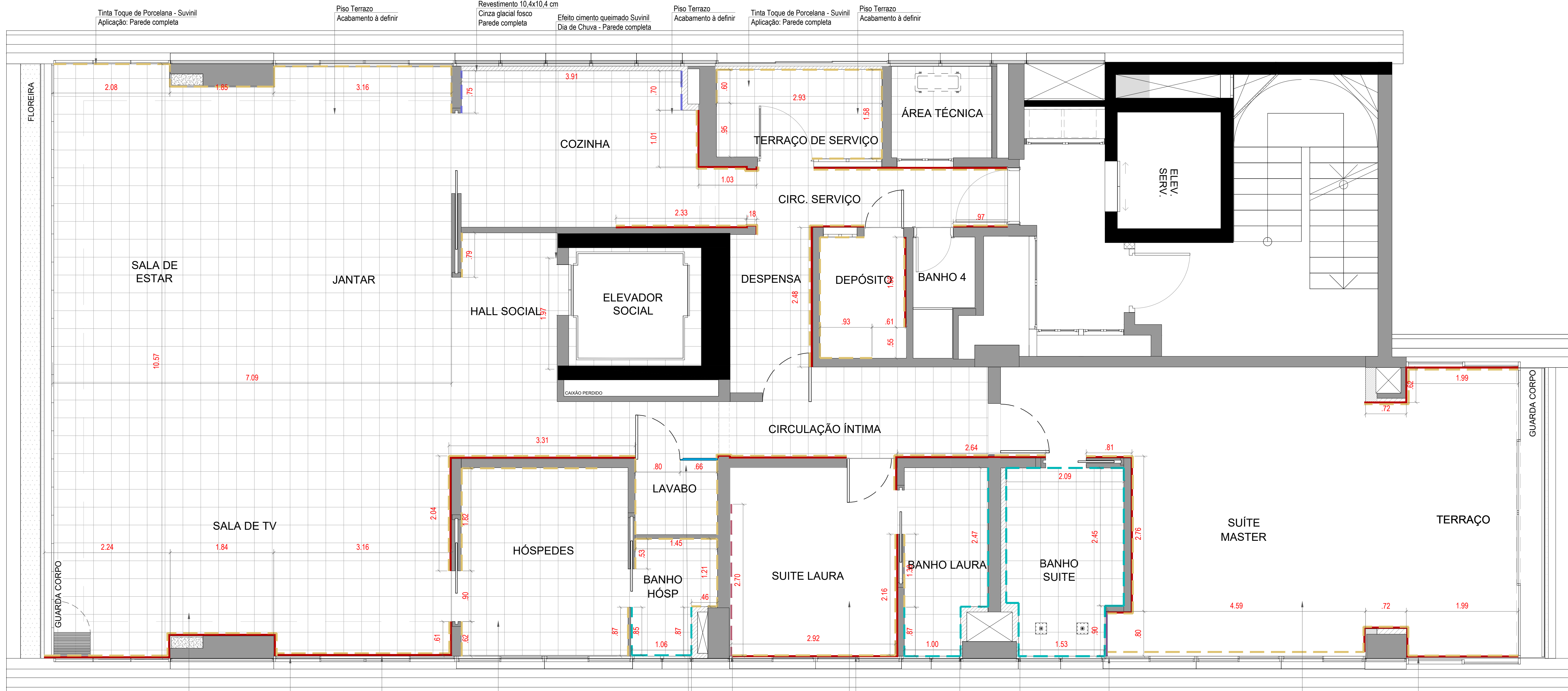
PLANTA PISO E REVESTIMENTOS AMBIENTE ESCALA 1:50
